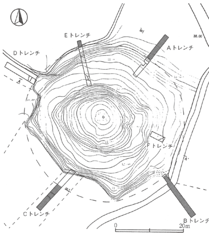
墳丘測量図
